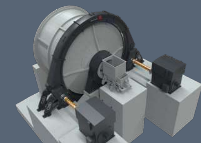
Entraînement QUADREX® pour les grands broyeurs SAC & Ball à partir de 20MW
